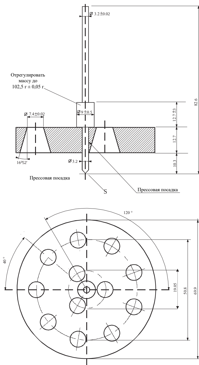
Рис. 1: Пенетрометр
